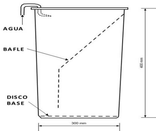
Figura 1. Recipiente para granular
