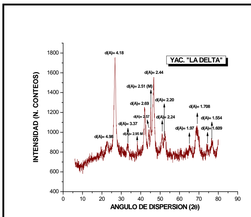
Figura 4. Difractograma de una muestra del horizonte limonítico (LB) del yacimiento “La Delta” en Moa, en la que predomina el oxihidróxido goethita, observándose además presencia de la espinela maghemita (M) y material amorfo.
