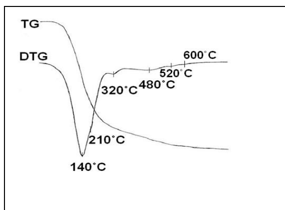
Figura 16. Termogramas TG y TGD de la muestra tecnológica (tipo III) de la arcilla niquelífera nontronítica del Peniplano Camagüey con presencia de goethita (-) 320 o C, muy poca montmorillonita (-) 520 o C, y trazas de serpentina (-) 600 o C.
