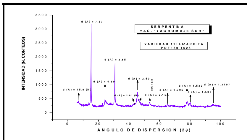
Figura 3. Difractograma de una muestra de serpentina (variedad lizardita, politipo 1T) del horizonte saprolítico del yacimiento “Yagrumaje Sur” en Moa. Se observa en ella poca arcilla nontronítica.
