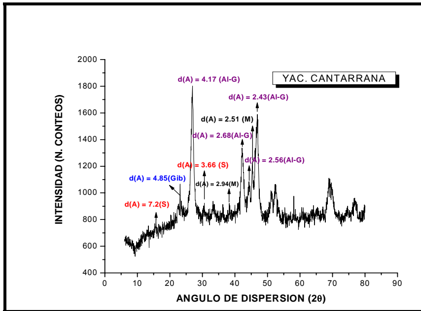
Figura 5. Difractograma de una muestra del horizonte limonítico del yacimiento “Cantarrana” (Moa), en la que predomina el oxihidróxido alumogoethita y presencia de la espinela magnetita (M), serpentina (S) material amorfo.
