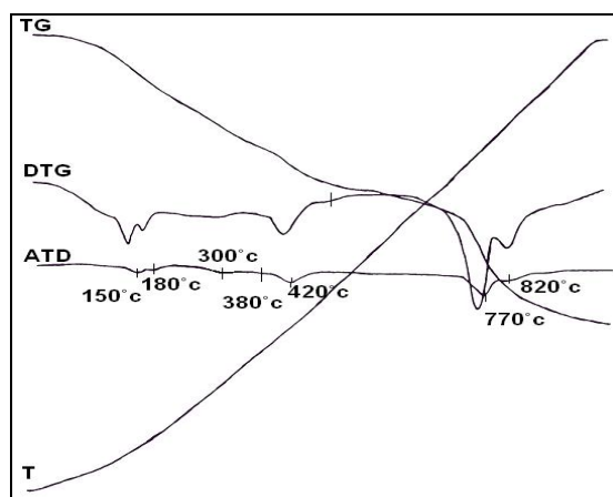
Figura 20. Termogramas ATD, TG y DTG de una muestra de residuo del proceso HPAL con presencia de mezclas de sulfatos: yeso (-) 1500C y 180 0 C; (-) 300 0 C goethita; jarosita (-) 420 0 C y (-) 770 0 C, alunita (-) 490 0 C y 820 0 C.
