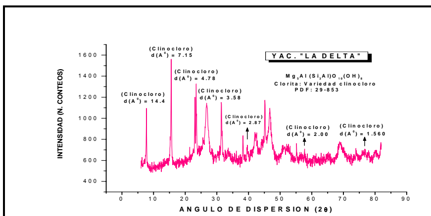
Figura 10. Difractograma de una muestra enriquecida en la arcilla clorita (variedad clinocloro) del yacimiento “Cantarrana” en Moa con presencia de goethita, espinela (maghemita) y gibbsita.
