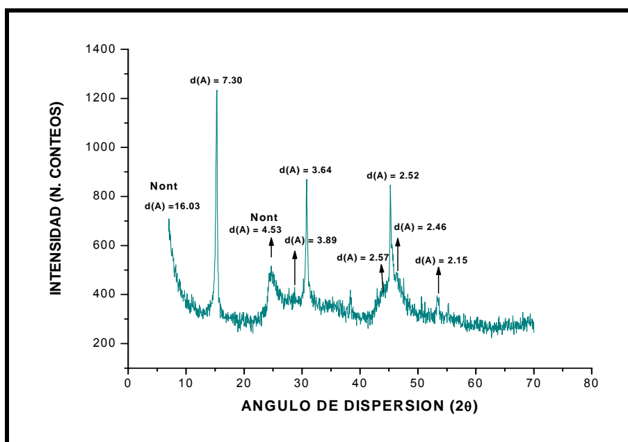
Figura 2. Difractograma de una muestra de serpentina variedad lizardita, con presencia además de la arcilla esmectítica nontronita de la zona de nontronitización del “Peniplano Camagüey”
