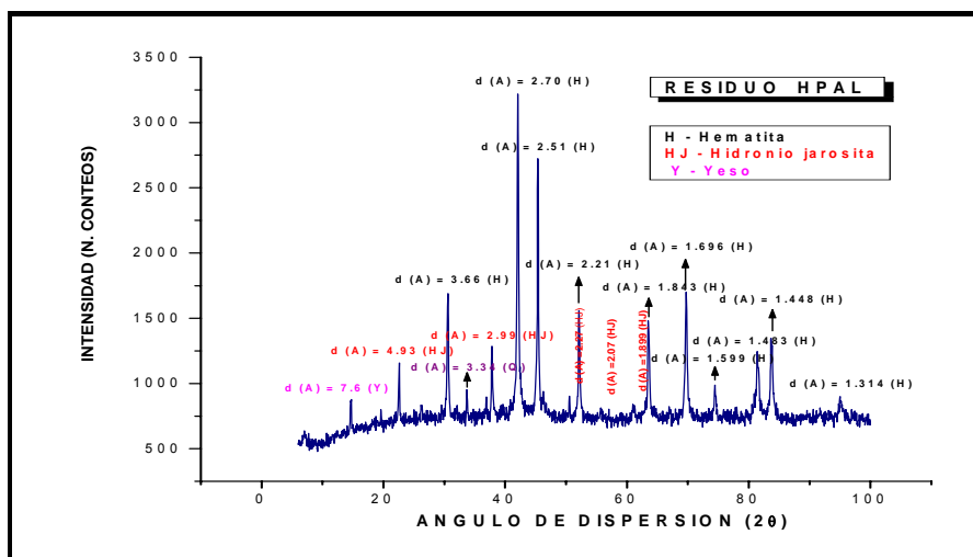
Figura 7. Difractograma del residuo del proceso HPAL de la Empresa “Pedro Soto Alba” (Moa) con presencia de hematita, sulfatos y trazas de cuarzo.
