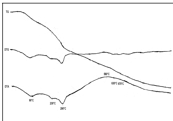
Figura 21. Termogramas ATD, TG y DTG de una muestra del Peniplano Camagüey con presencia de mezclas de: ernieniquelita (-) 230 o C; goethita (-) 290 o C; (+) 580, 630 y 670 o C de mezclas de espinelas magnetita y trevorita.
