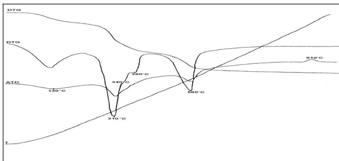
Figura 14. Termogramas ATD -TGD -TG de una muestra del horizonte limonítico -ocre inestructural- del depósito “Yagrumaje Norte” en Moa, donde se aprecia un sistema contiguo de efectos térmicos en forma de hombros y característicos de las especies: goethita (-) 310°C; gibbsita (-) 340°C; 380°C (20% Al iónico) y la arcilla caolinítica halloysita (-) 560°C y (+) 910°C
