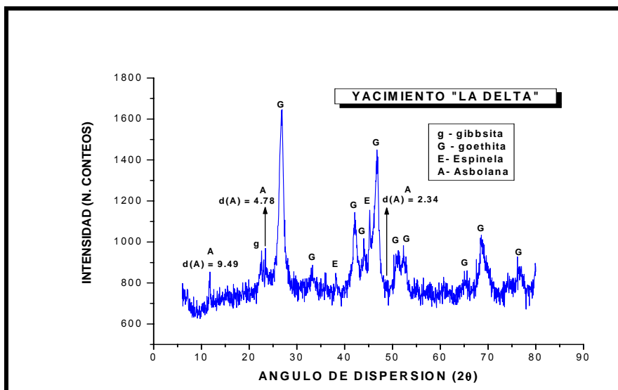
Figura 8. Difractograma de una muestra de ocre estructural correspondiente al horizonte limonítico del yacimiento “La Delta” en Moa con presencia del mineral de Mn (asbolana), goethita y espinela (maghemita).
