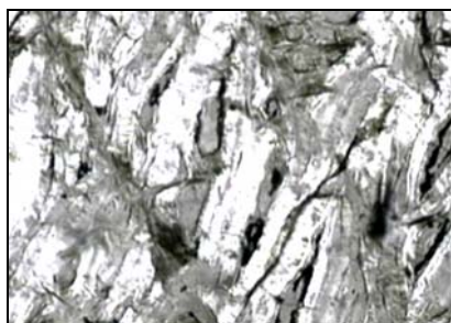
Figura 23. Hojuelas de serpentina antigorítica con placas de Lizardita, Nicles II.
