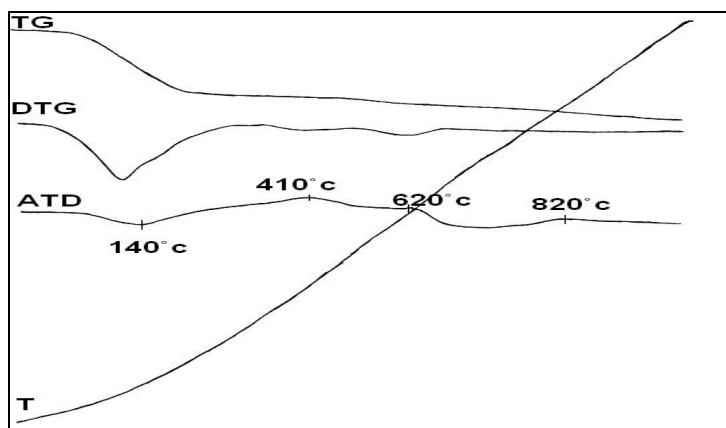
Figura15. Termogramas ATD-TGD -TG de una muestra de residuo del proceso CARON, en el que se aprecia el sistema de efectos exotérmicos característicos de las espinelas de Fe (magnetita-maghemita) y/o Fe-metal (cromita y trevorita); (+) 410°C y (+) 820°C.
