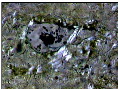
Figura 22. Gránulos amorfos de Serpofita (Se), rodeados de Antigorita (An), Clorita (Cl), Nicles II.
