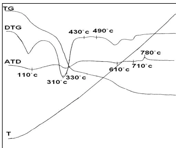
Figura 19. Termogramas ATD, TG y DTG del mineral de rechazo de Moa con predominio de goethita (-) 310°C, gibbsita (-) 330°C, asbolana (-) 430°C, nontronita (-) 490°C y mezclas de serpentinas: crisotilo (-) 610°C; (+) 780°C y antigorita (-) 710°C.
