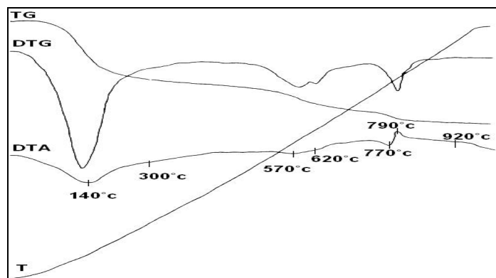
Figura 17. Termogramas ATD, TG, DTG de una muestra correspondiente al horizonte de arcilla ocrosa del yacimiento “Yagrumaje Norte” Moa con presencia de: clorita: (-) 620^{\circ}\text{C} ; (-) 770^{\circ}\text{C} ; (+) 790^{\circ}\text{C} , caolinita -variedad halloysita- (-) 140^{\circ}\text{C} ; (-) 570^{\circ}\text{C} ; (+) 920^{\circ}\text{C} , y muy poca goethita (-) 300^{\circ}\text{C} .
