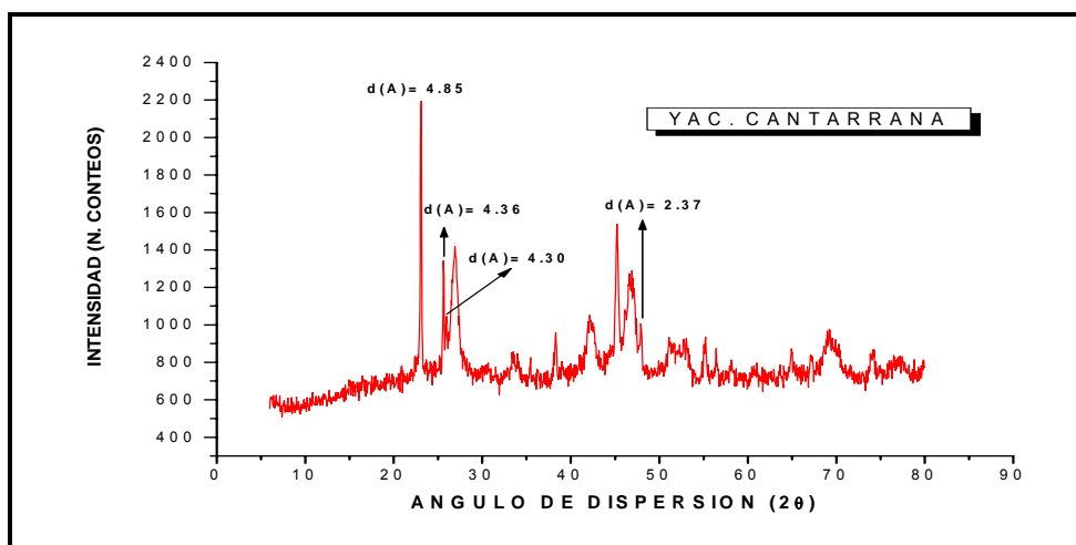
Figura 12. Difractograma de una muestra correspondiente al horizonte limonítico enriquecida con el mineral gibbsita (yacimiento “Cantarrana”, región de Moa).
