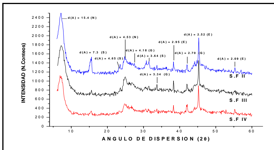
Figura 11. Difractogramas de polvos de rayos-X de muestras del Peniplano Camagüey con nontronita (fase principal), acompañada de serpentina, goethita y la espinela Fe-Ni trevorita
