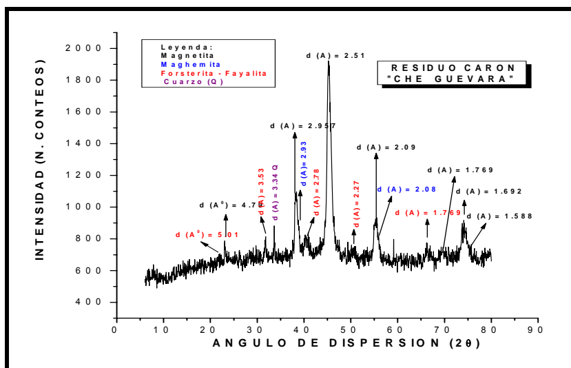
Figura 6. Difractograma del residuo industrial del proceso CARON de la Empresa “Che Guevara”(Moa) donde se observa presencia abundante de mezclas de espinelas de hierro magnetitmaghemita como fases mayoritarias.
