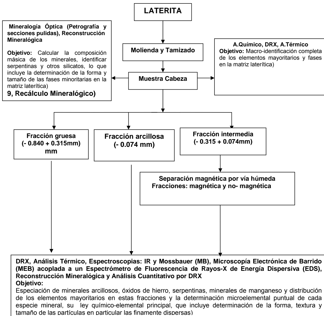
Figura 1. Esquema de preparación y procedimientos analíticos que se proponen para ejecutar los estudios de composición sustancial de las menas lateríticas cubanas.
