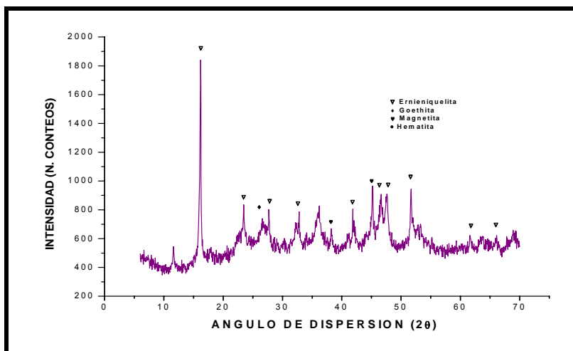
Figura 9. Difractograma de polvos DRX de la fracción (-0.840 + 0.074mm) de una muestra tecnológica del Peniplano Camagüey, donde se reportó por primera vez en el país el mineral de manganeso Ernieniquelita ( NiMn_3O_7 \cdot 3H_2O )
